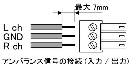
[図 8.11] ターミナルブロック (3 ピン) へのオーディオケーブルの接続方法
