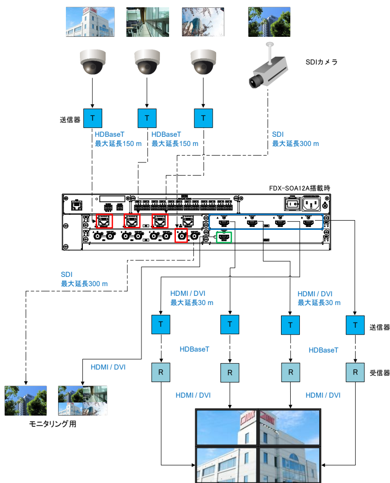
[図 8.1] 映像機器の接続 (図 : FDX-S08U)
