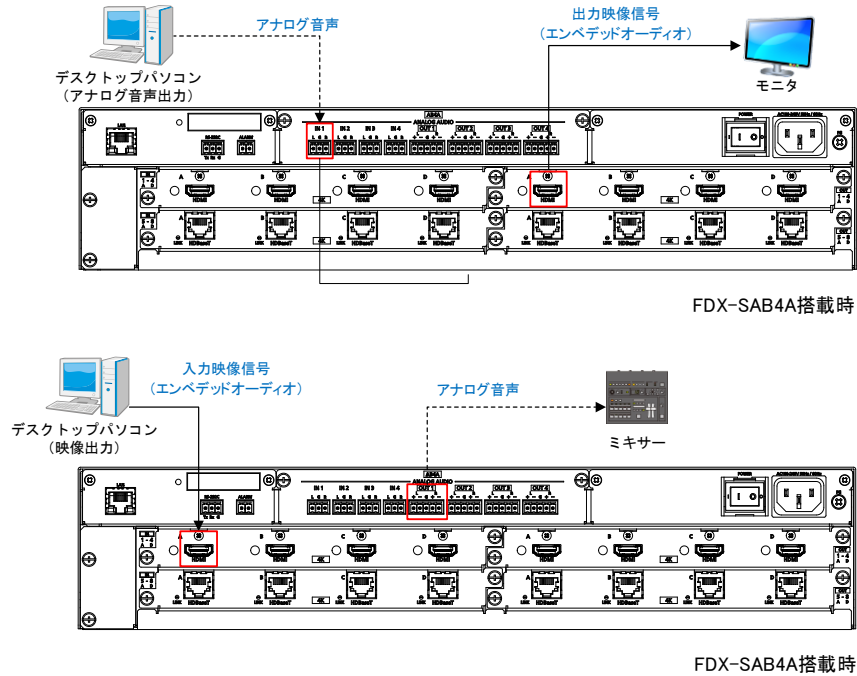
[図 8.6] 音声機器の接続 (図 : FDX-S08U に FDX-SAB4A 搭載)
