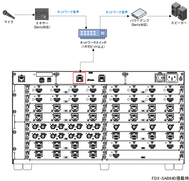
[図 8.7] 音声機器の接続 (図 : FDX-S32U に FDX-SAB64D 搭載)
