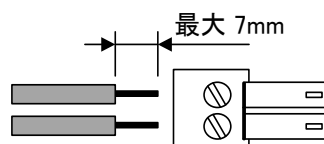
【図 8.5】ターミナルブロック (2 ピン) へのケーブルの接続方法
