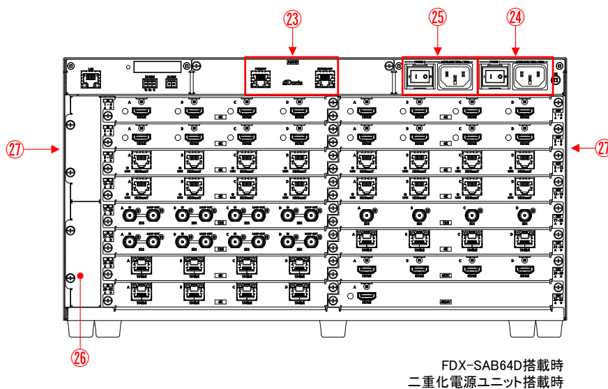
[図 5.3] 外観図
