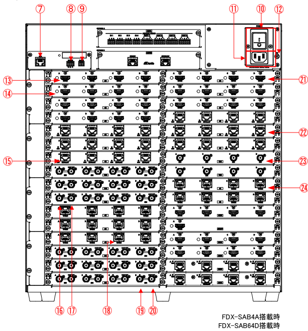
[図 5.4] 外観図
