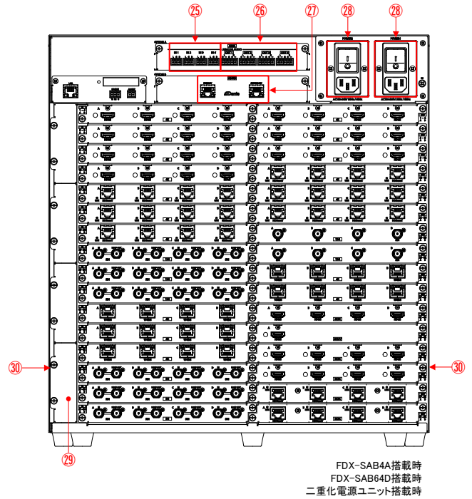
[図 5.4] 外観図
