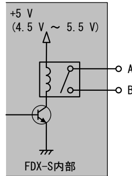
[図 10.48] アラーム出力回路
