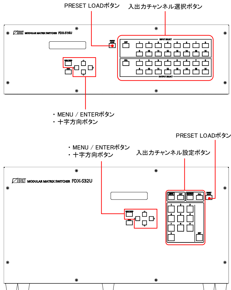
【図 9.3】 ボタンロックの対象 (上：FDX-S16U、下：FDX-S32U)
