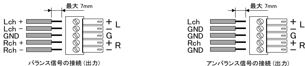
[図 8.10] ターミナルブロック (5 ピン) へのオーディオケーブルの接続方法
