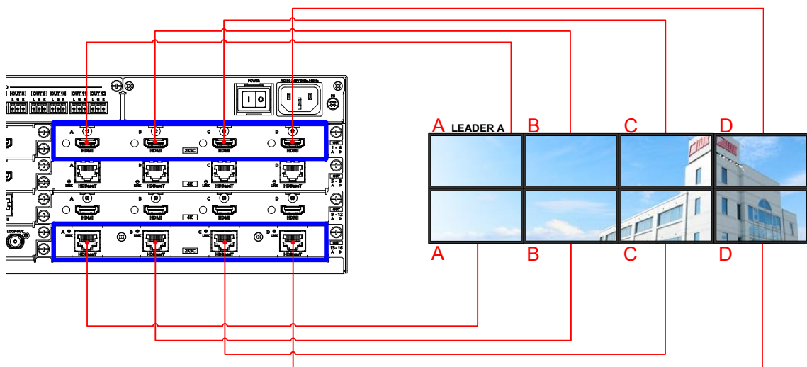
[図 10.12] 同期設定 (スロットが離れた場合の4×2画面)
