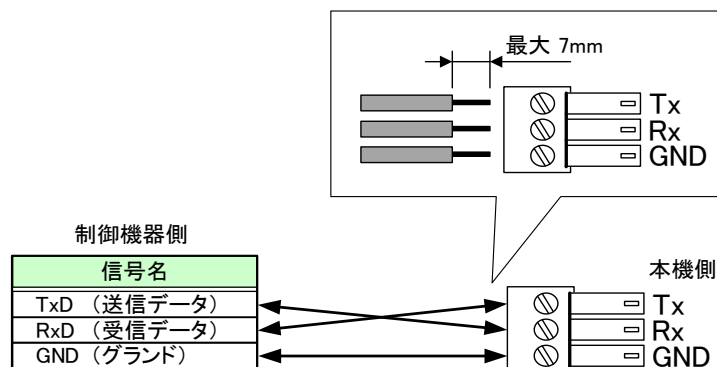
[図 8.4] ターミナルブロック (3 ピン) へのケーブルの接続方法
