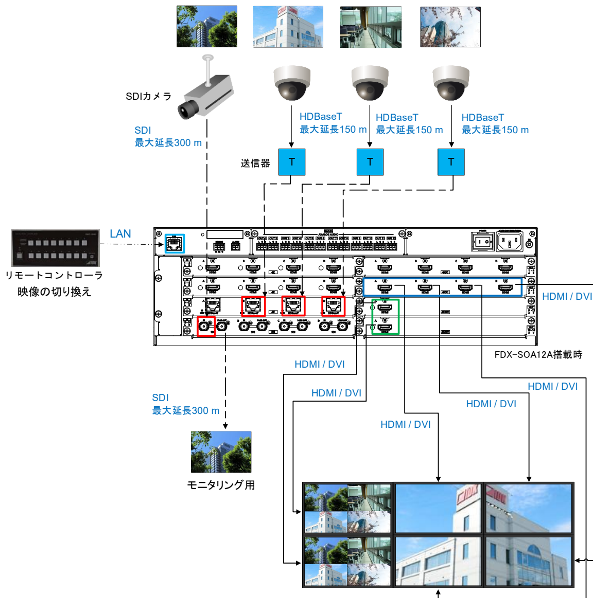
[図 6.1] システム構成例 (図 : FDX-S16U)
