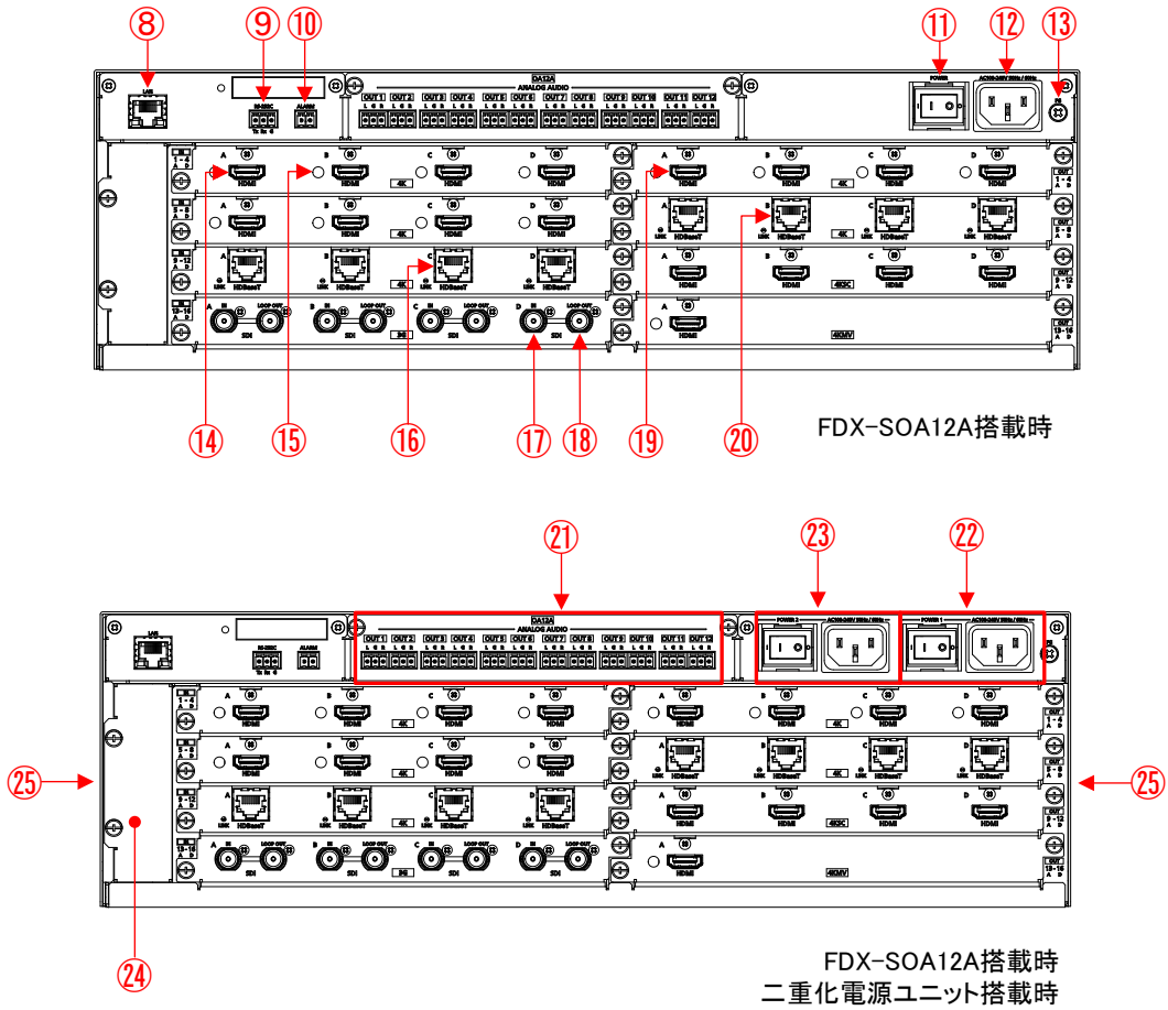
[図 5.2] 外観図
