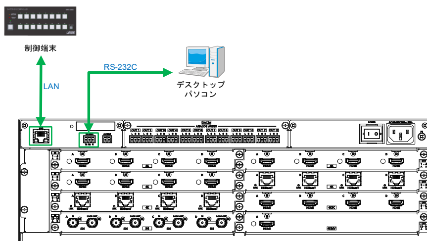
[図 8.3] 制御機器の接続 (図 : FDX-S16U)
