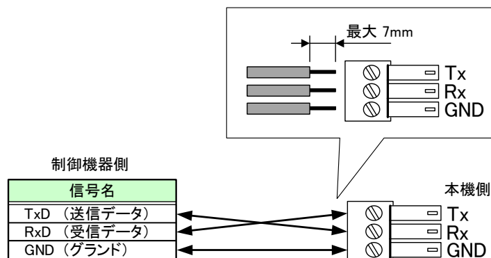
[図 2.1] ターミナルブロック (3 ピン) への RS-232C ケーブルの接続方法
