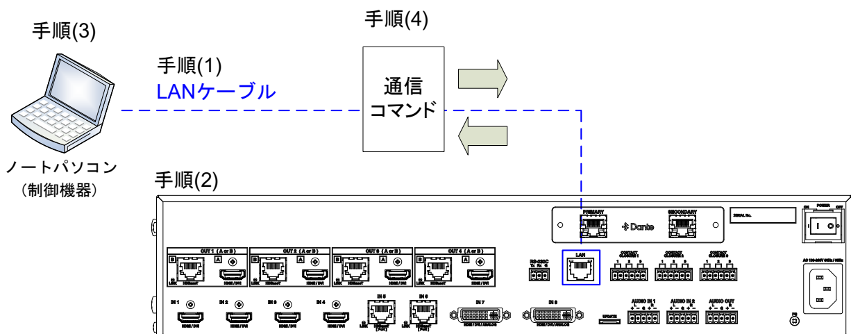
[図 2.4] LAN 通信による制御
