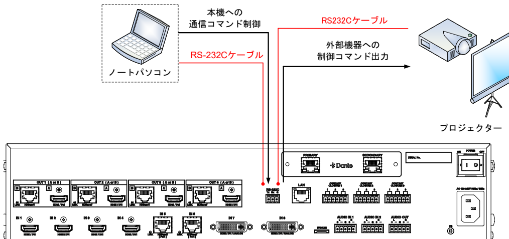
[図 2.2] RS-232C 通信の動作例
