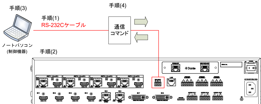
[図 2.1] RS-232C 通信の設定手順
