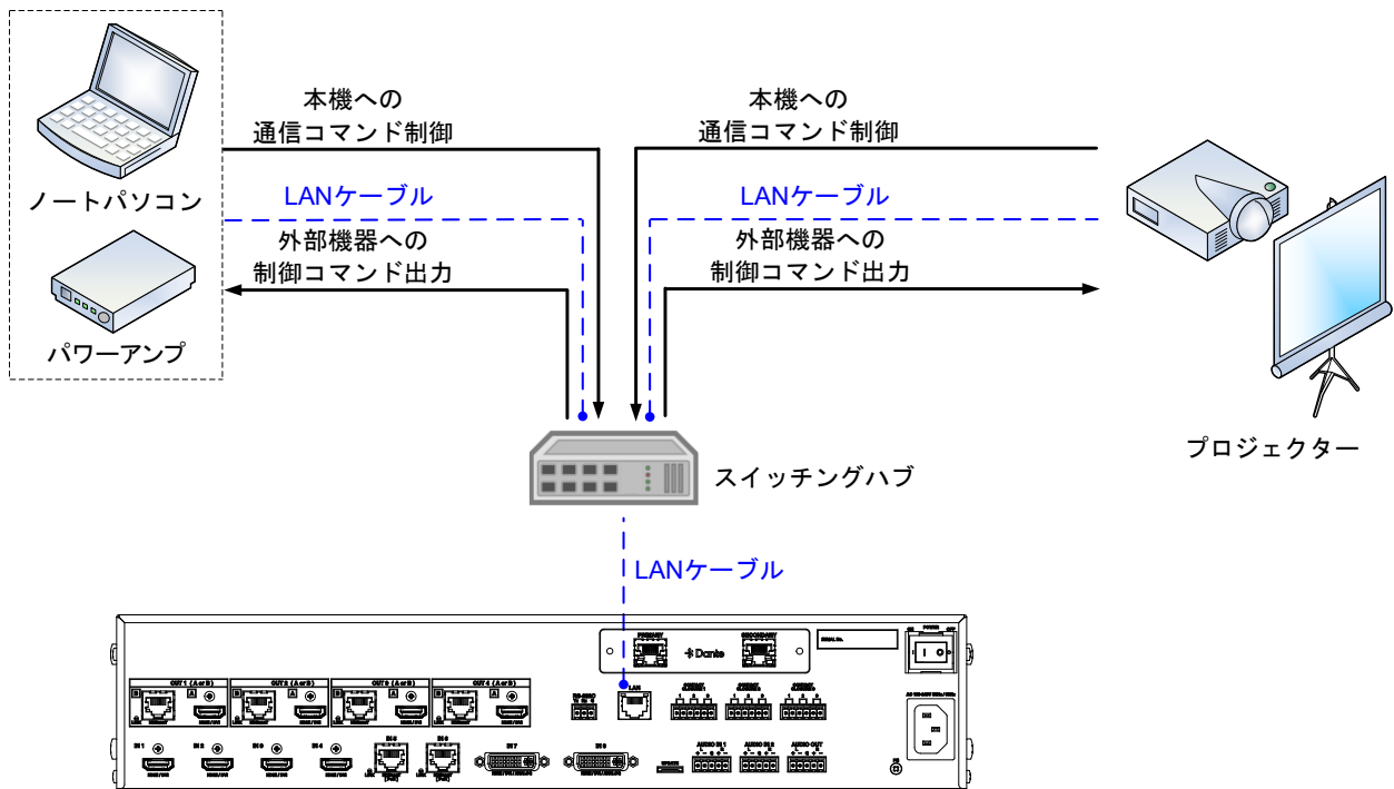
[図 2.5] LAN 通信の動作例
