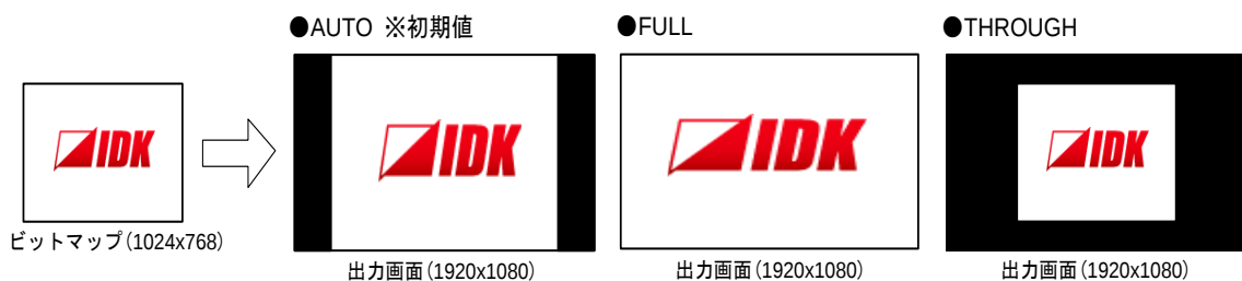
[図 9.35] アスペクト比設定
