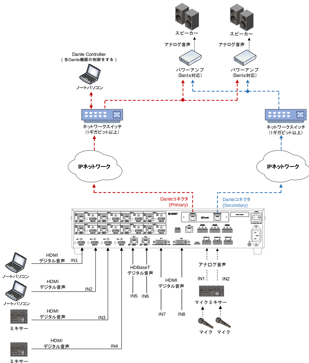
【図. 8.15】 二重化接続
