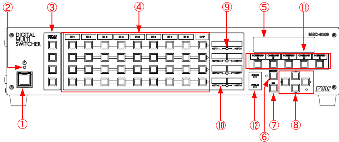
[図 5.1] フロントパネルの外観図 (図 : MSD-6208)
