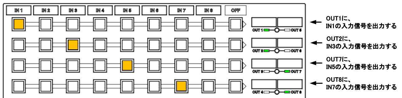
[図 8.2] 入出力チャンネルの設定(図:MSD-6208)
