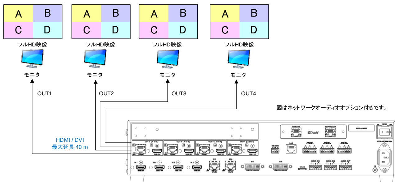
[図 8.4] 合成モード時の映像出力例 (図 : MSD-6204)
