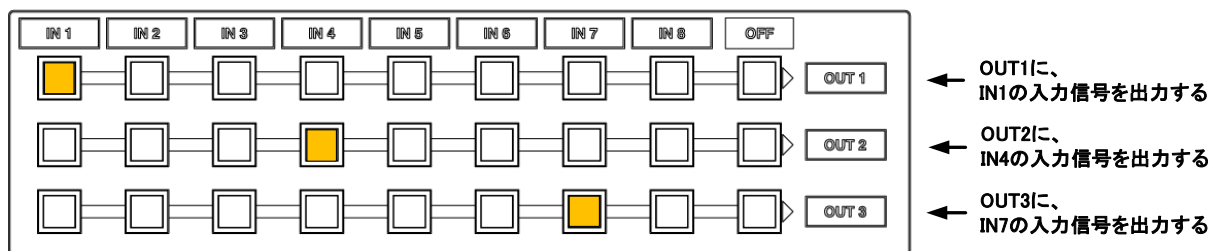
[図 8.1] 入出力チャンネルの設定(図:MSD-6203)
