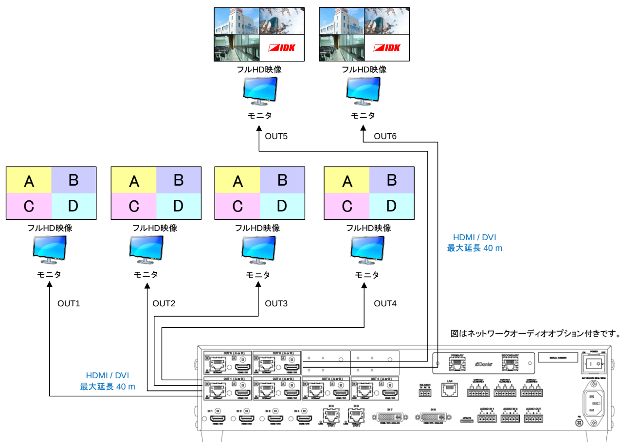
[図 8.5] 合成モード時の映像出力例 (図 : MSD-6206)
