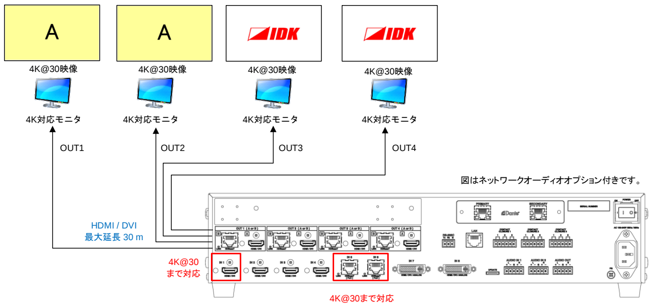
[図 8.10] 4K モード時の映像出力例 (図 : MSD-6204)
