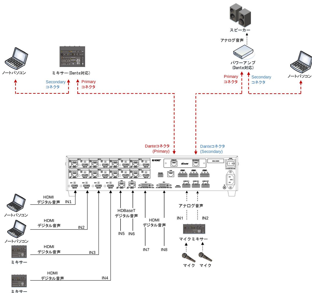
[図. 8.16] デイジーチェーン接続
