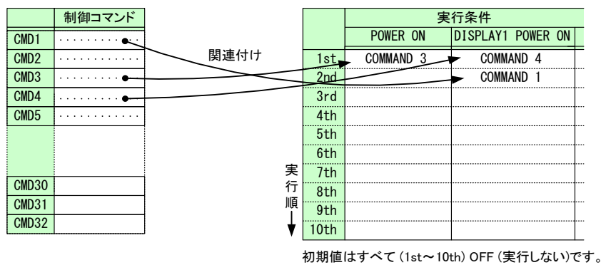
[図 9.31] 制御コマンドの関連付け
