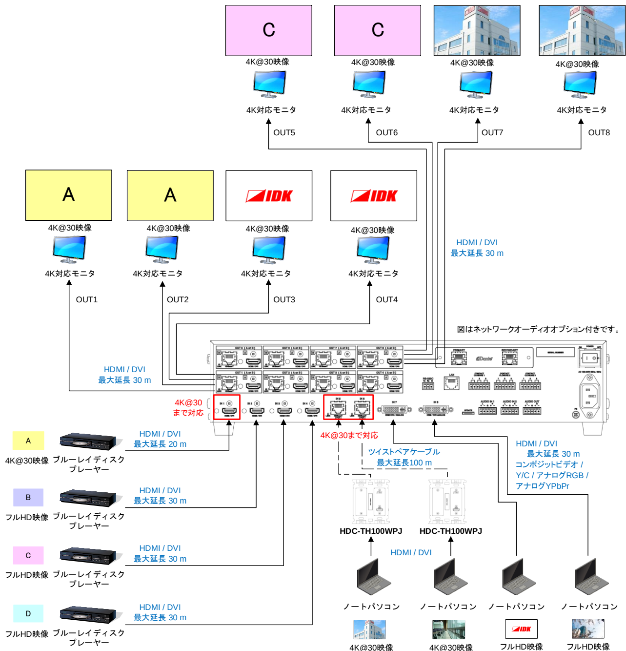
[図 6.3] 4K モードのときの接続例 (図 : MSD-6208)
