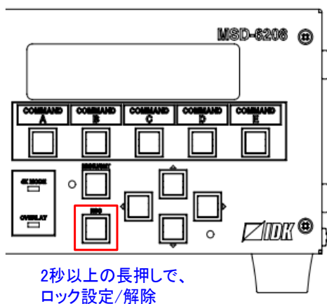
[図 8.14] エスケープボタンによるロック設定／解除 (図 : MSD-6208)
