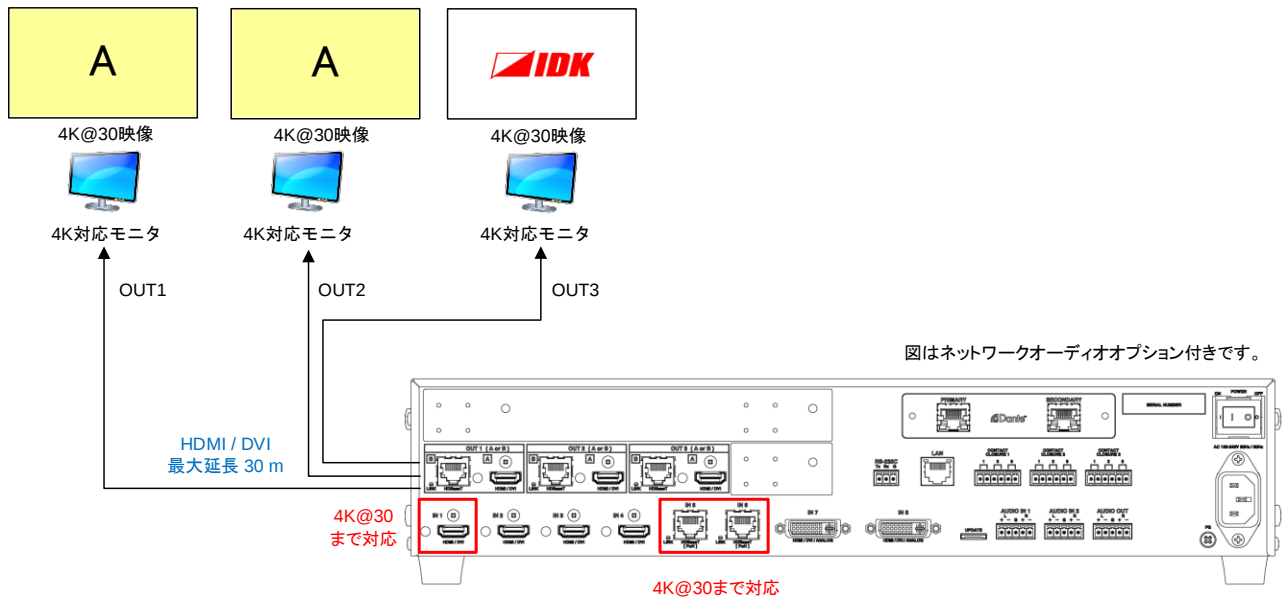
[図 8.9] 4K モード時の映像出力例 (図 : MSD-6203)
