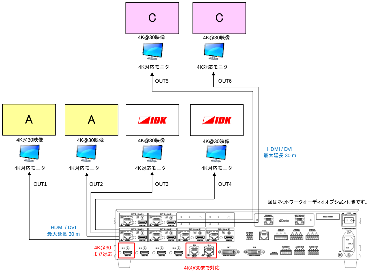
[図 8.11] 4K モード時の映像出力例 (図 : MSD-6206)
