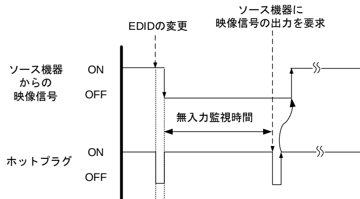
[図 9.14] 映像信号の無入力監視時間
