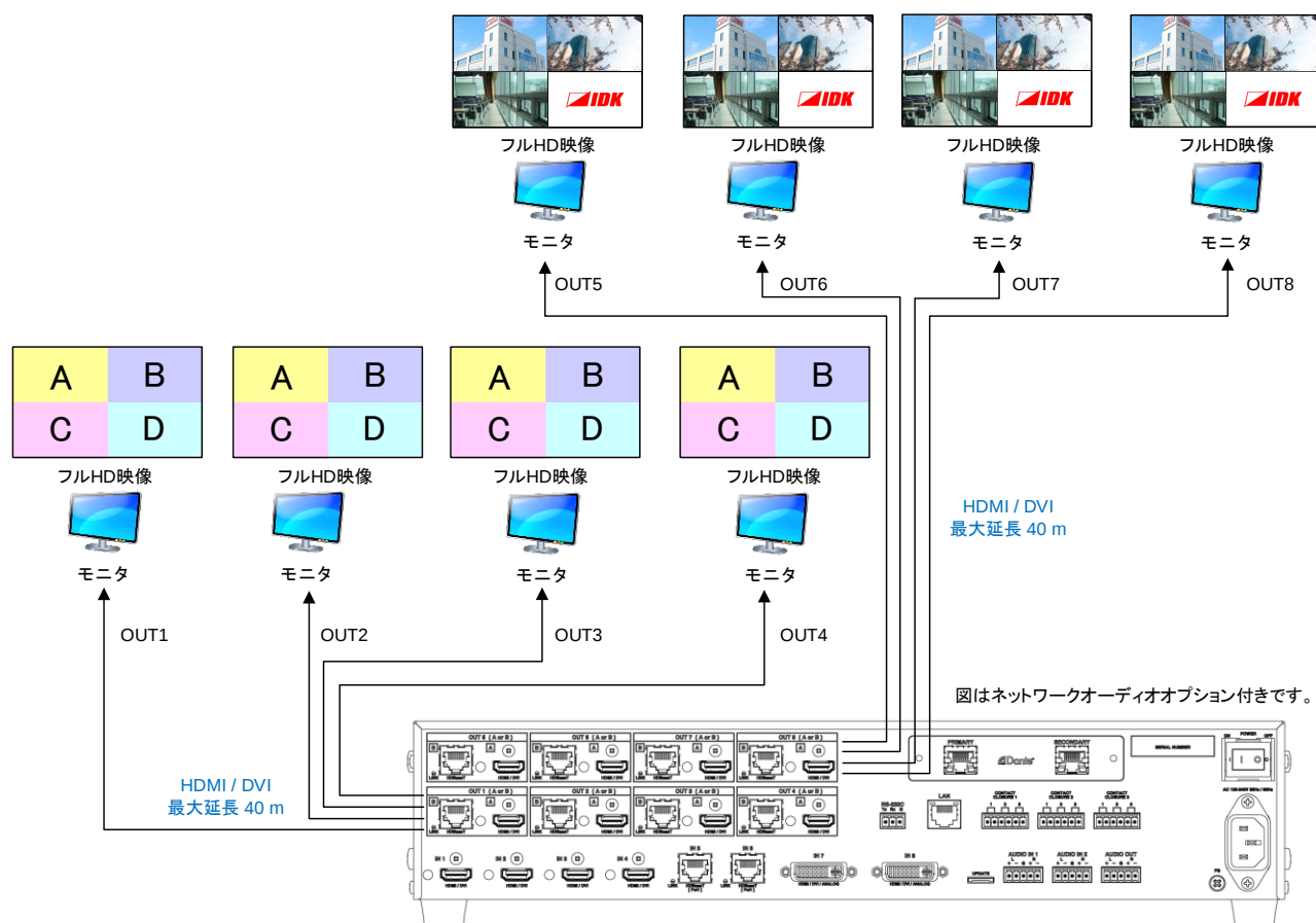
[図 8.6] 合成モード時の映像出力例 (図 : MSD-6208)
