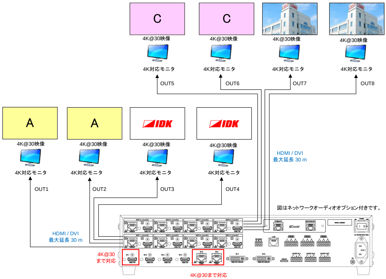
[図 8.12] 4K モード時の映像出力例 (図 : MSD-6208)
