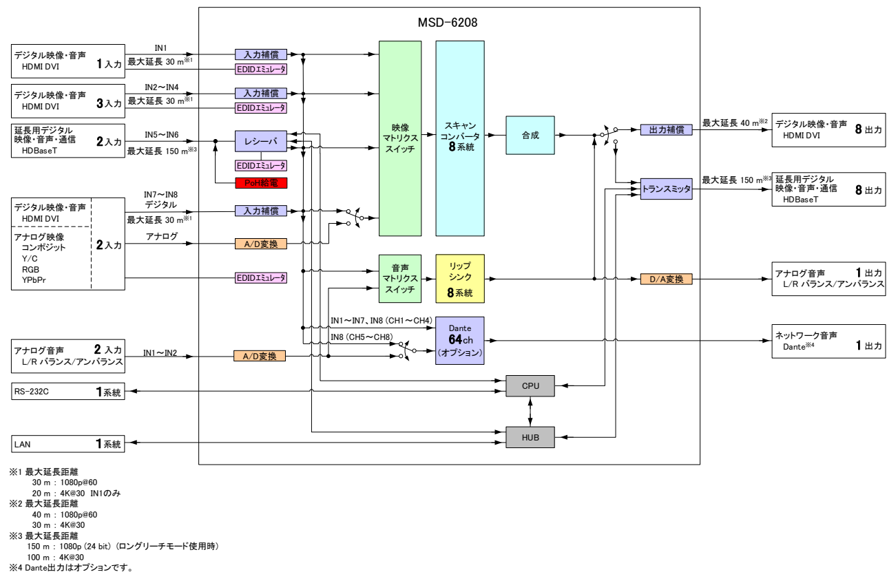
[図 3.1] MSD-6208 のブロック図
