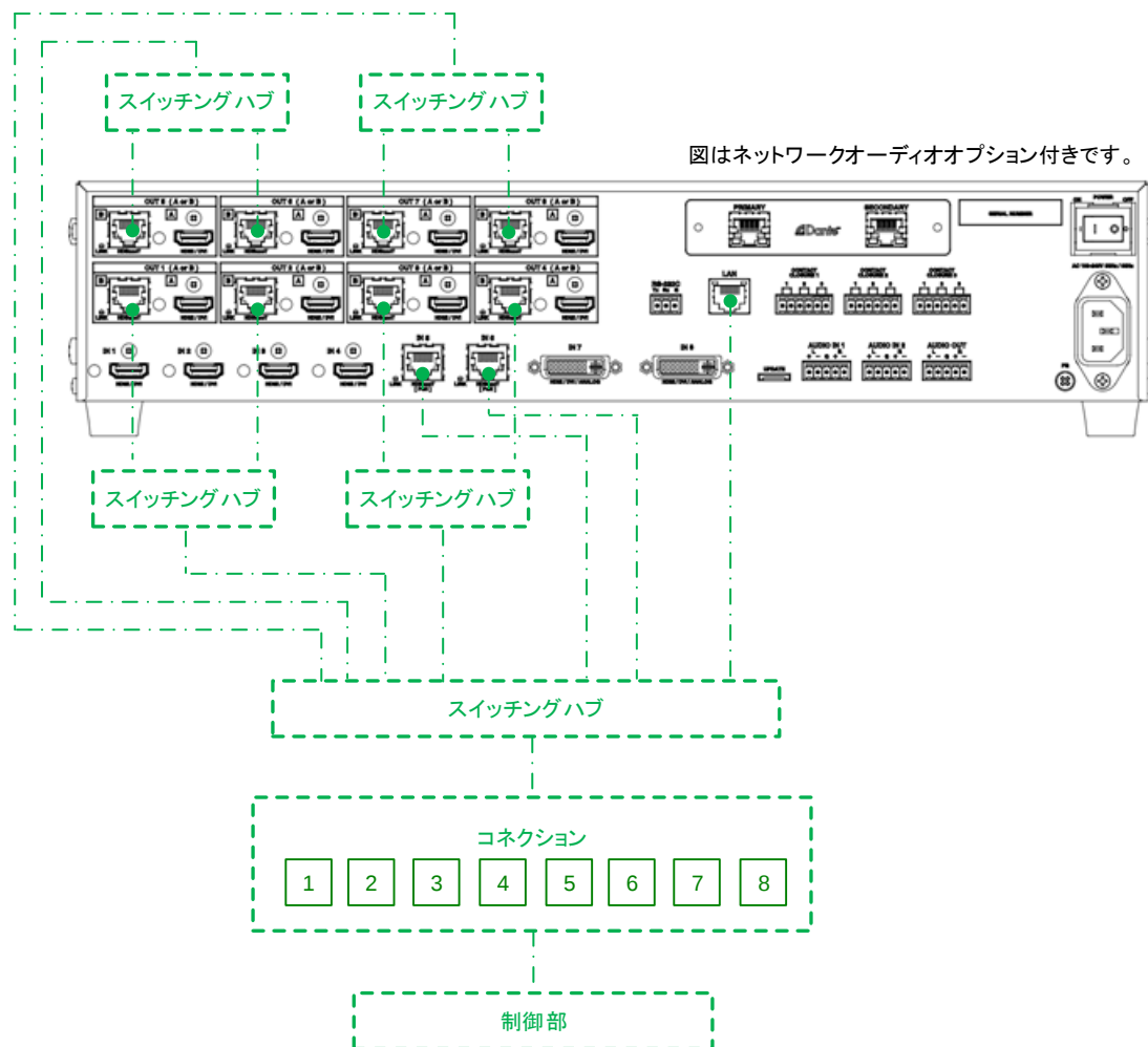
[図 9.27] 本機内部の LAN 機能構成 (図 : MSD-6208)
