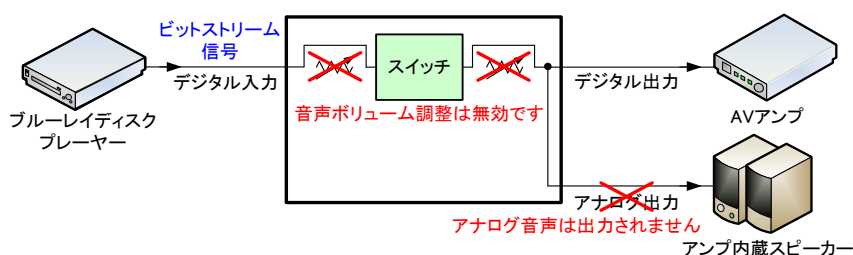
[図 9.23] ビットストリーム信号の入力
