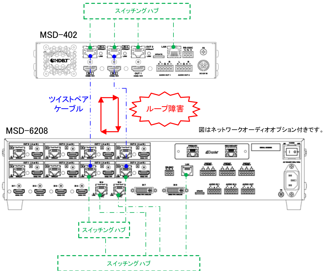
[図 9.28] IDK 製品を用いたループ障害例 (図 : MSD-6208)
