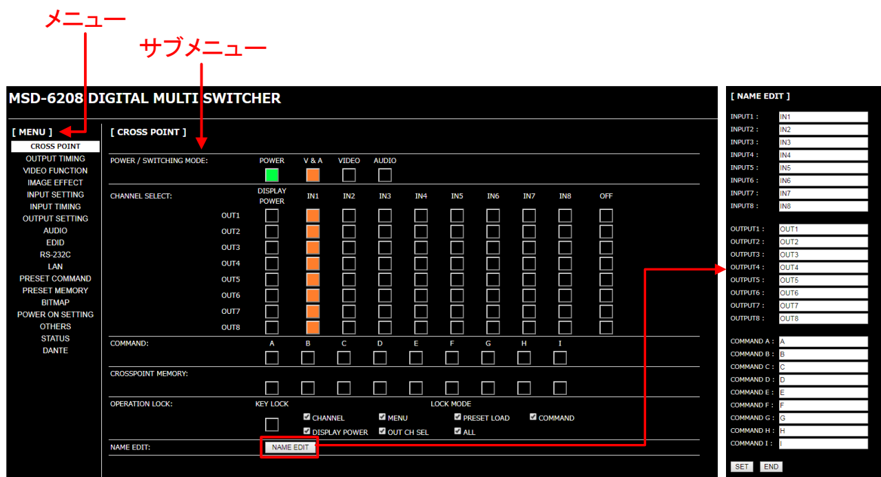
[図 8.17] WEB ブラウザからの制御画面
