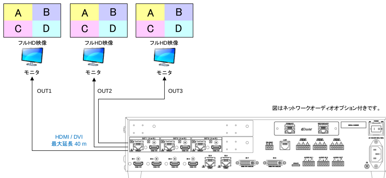
【図 8.3】 合成モード時の映像出力例 (図：MSD-6203)
